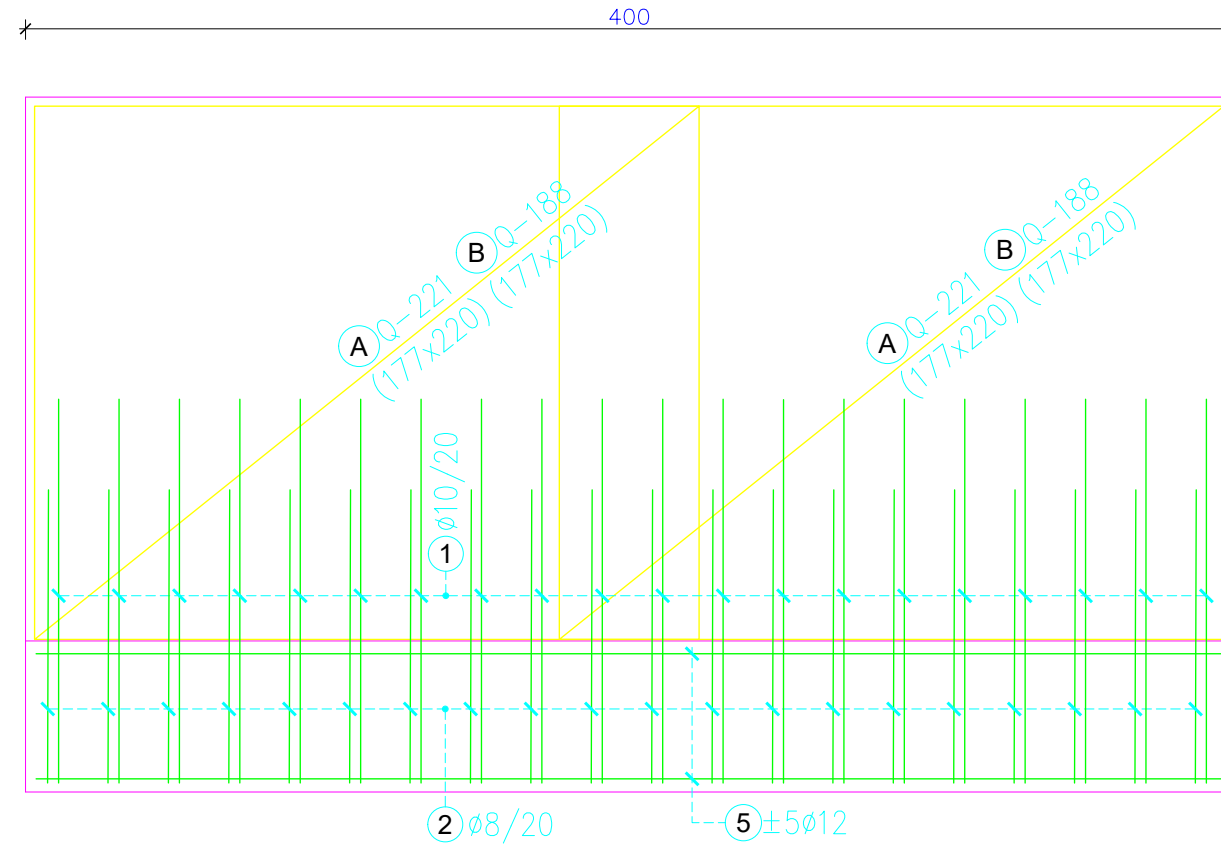
zid Z3 u pogledu
