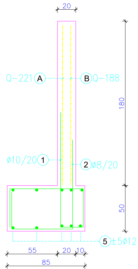
presjek zida Z3
