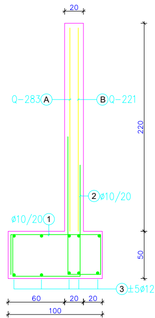
presjek zida
