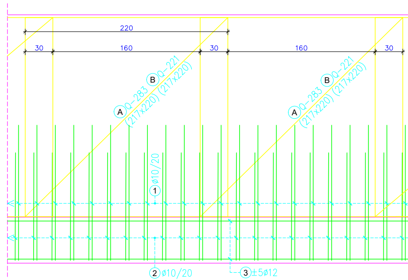
dio zida u pogledu (Lukupno=8,6 m)
